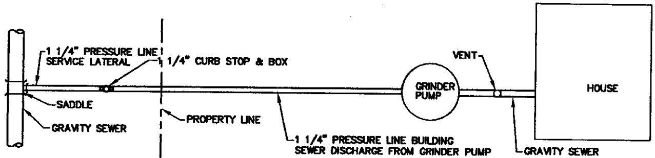
PLAN N.T.S.
