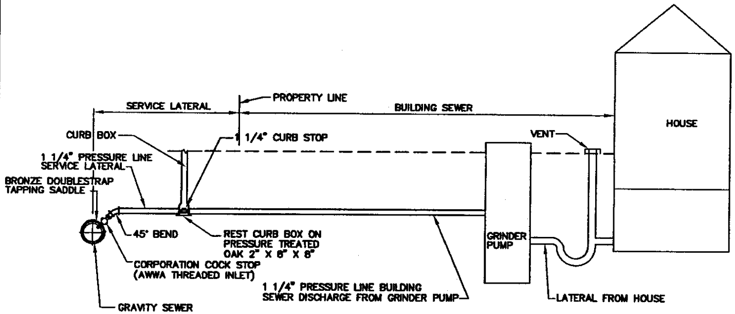
SECTION N.T.S.
