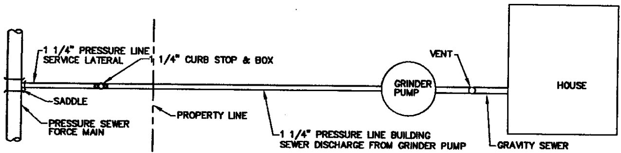
PLAN N.T.S.
