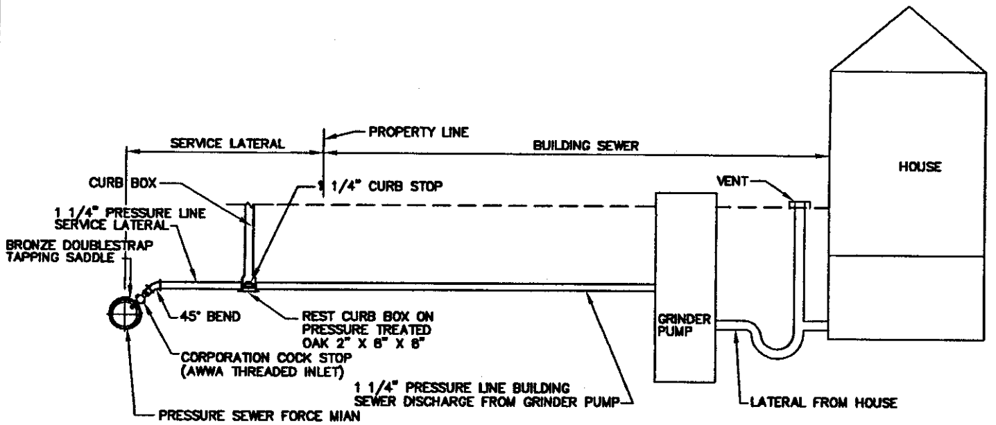
SECTION N.T.S.
