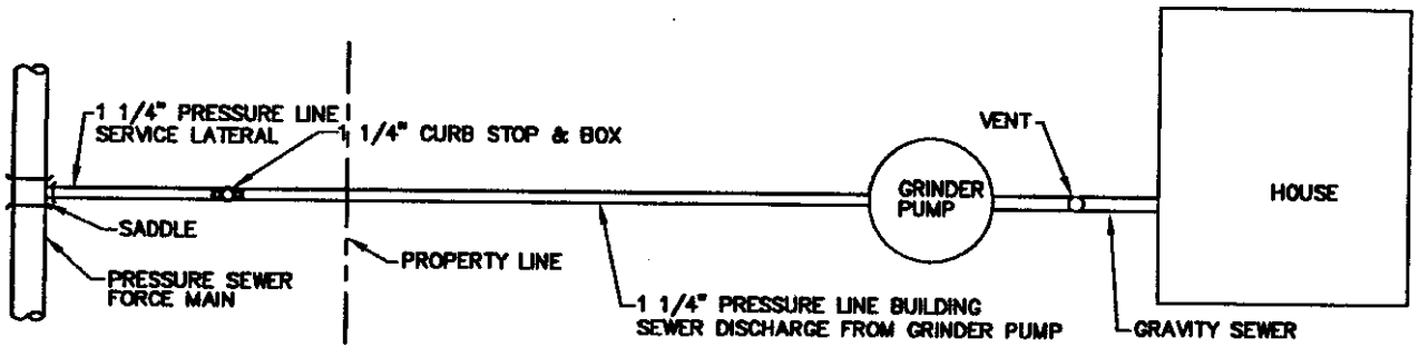
PLAN N.T.S.
